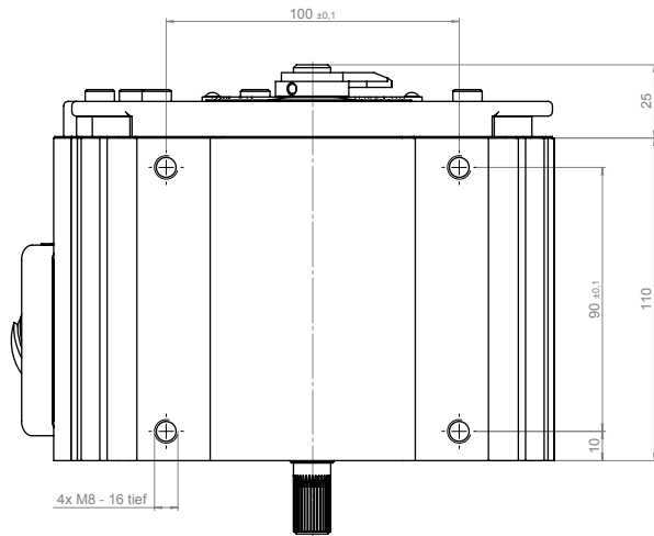
ANSICHT X
